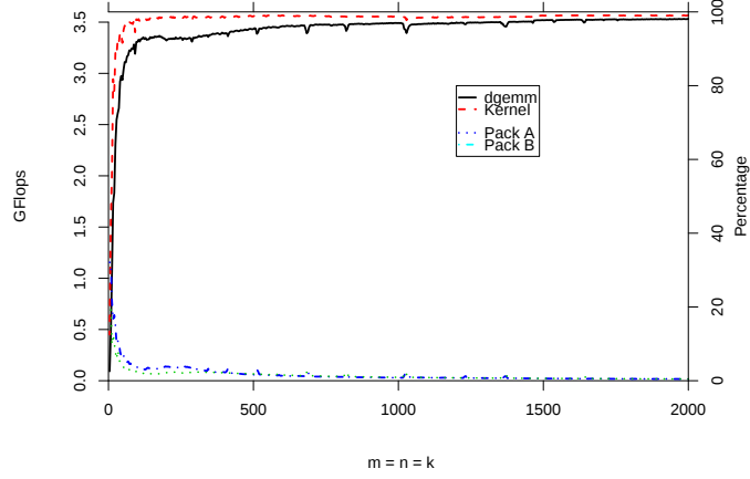
Fig. 17. Itanium2 (1.5 GHz).
